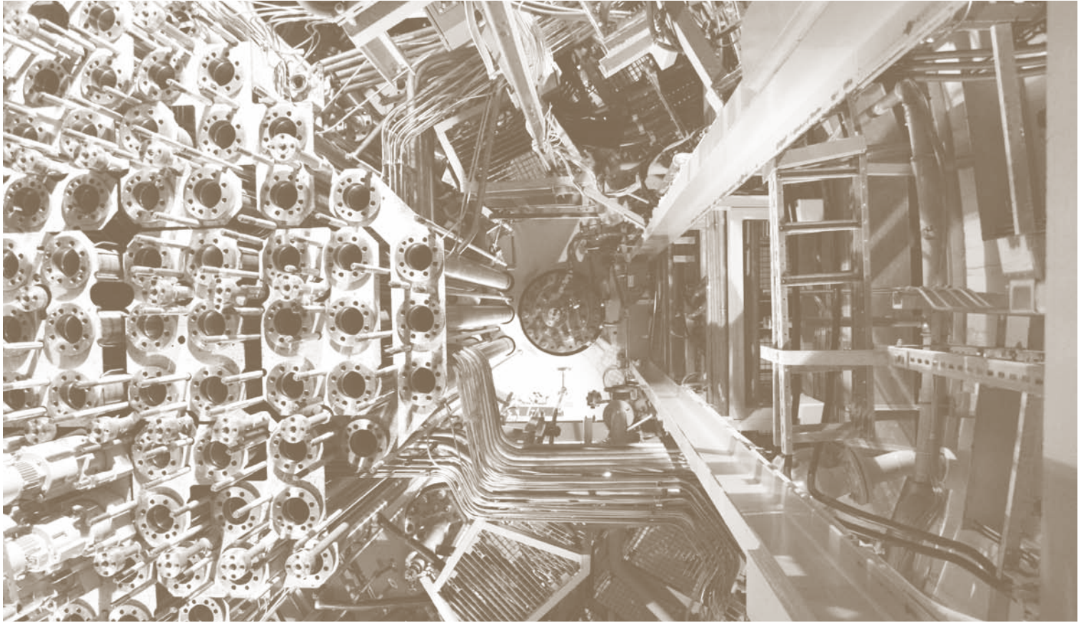
Brennstabsteuerung im Atomkraftwerk Zwentendorf/Österreich. Der Meiler aus den 1970er-Jahren ging nie in Betrieb. Fotos (3): Gnal/Flickr
